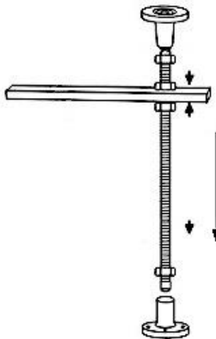
Крепление задней шпильки
